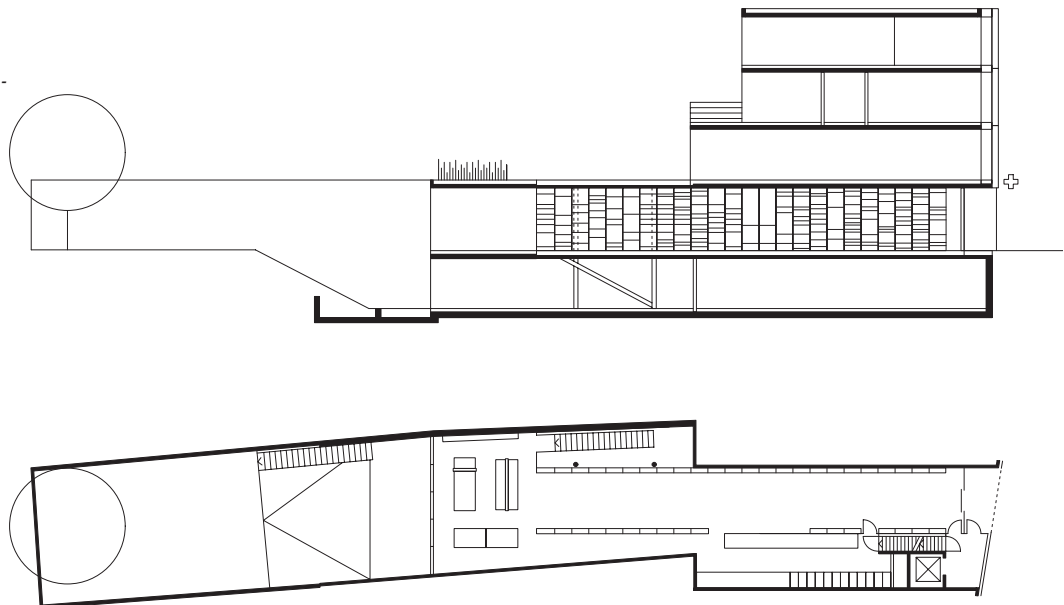
Schnitt, Grundriss Erdgeschoss M 1:400
